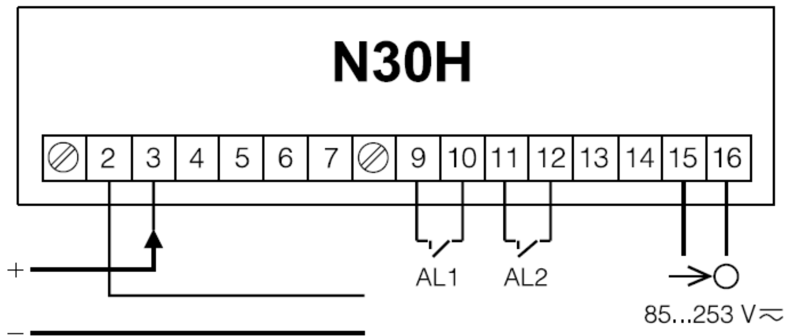
Рис.5. Схема электрических соединений измерительного прибора N30H для измерения тока
