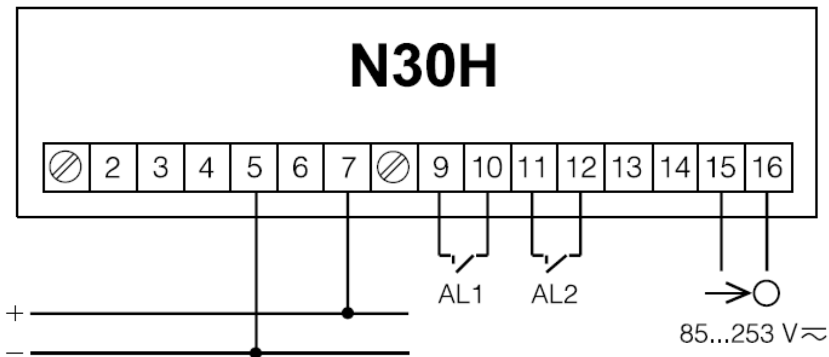
Рис.6. Схема электрических соединений измерительного прибора N30H для измерения напряжения
