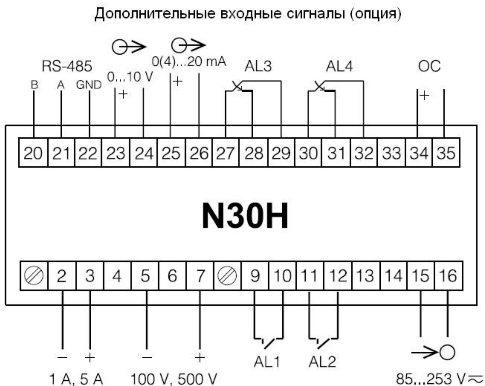
Рис. 4. Схема электрических соединений прибора N30H. Описание клеммного ряда
