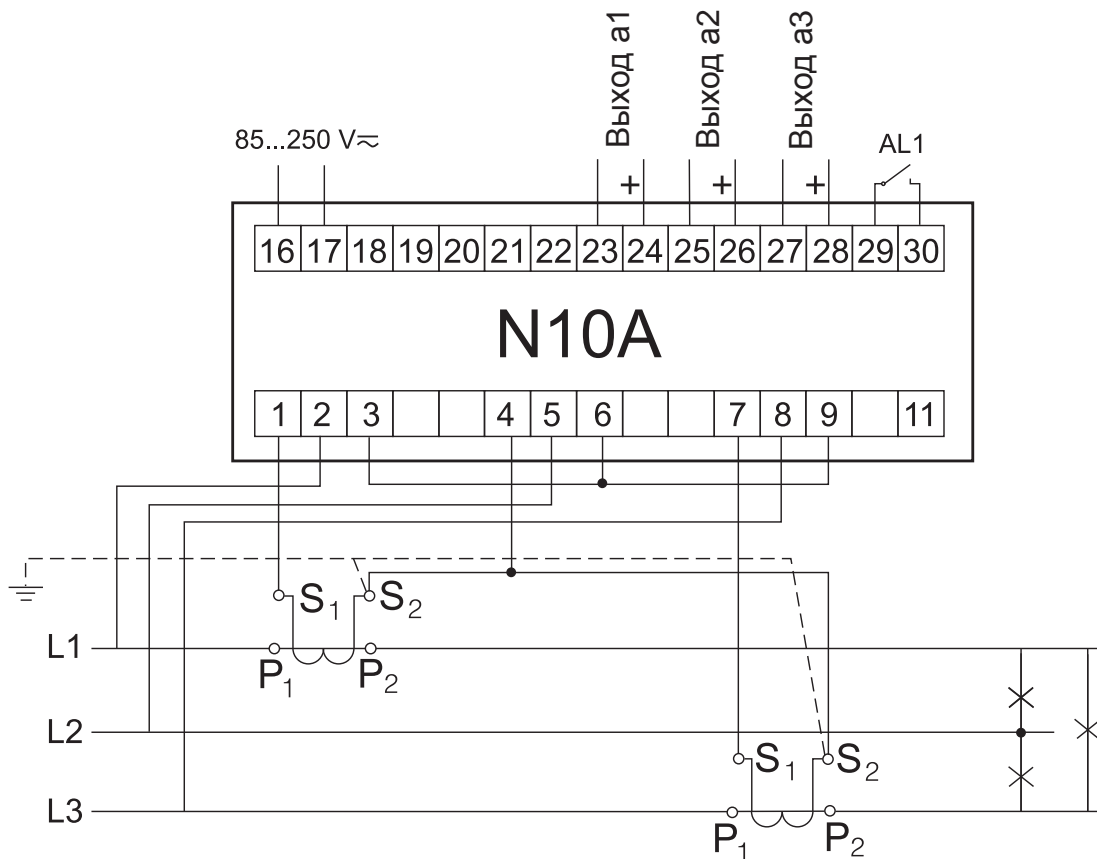
Прямое измерение в 3-проводной сети
