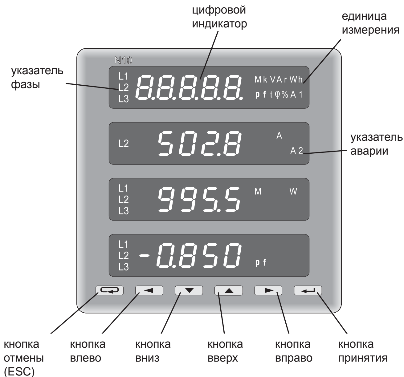
Рис. 5. Вид внешней панели прибора N10A.
