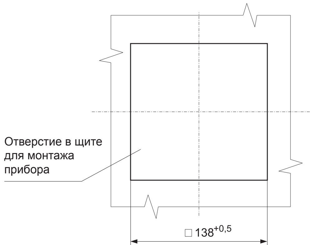
Рис.1. Размер отверстия и метод установки анализатора N10A.
