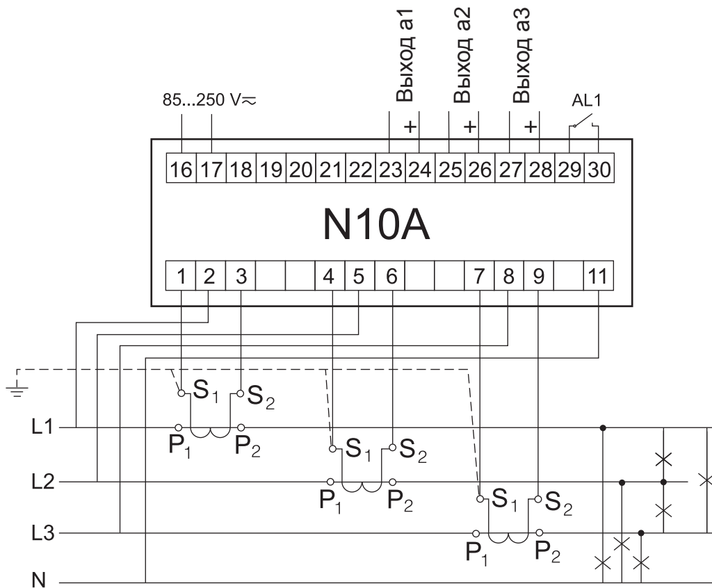
Полупрямое измерение в 4-проводной сети
