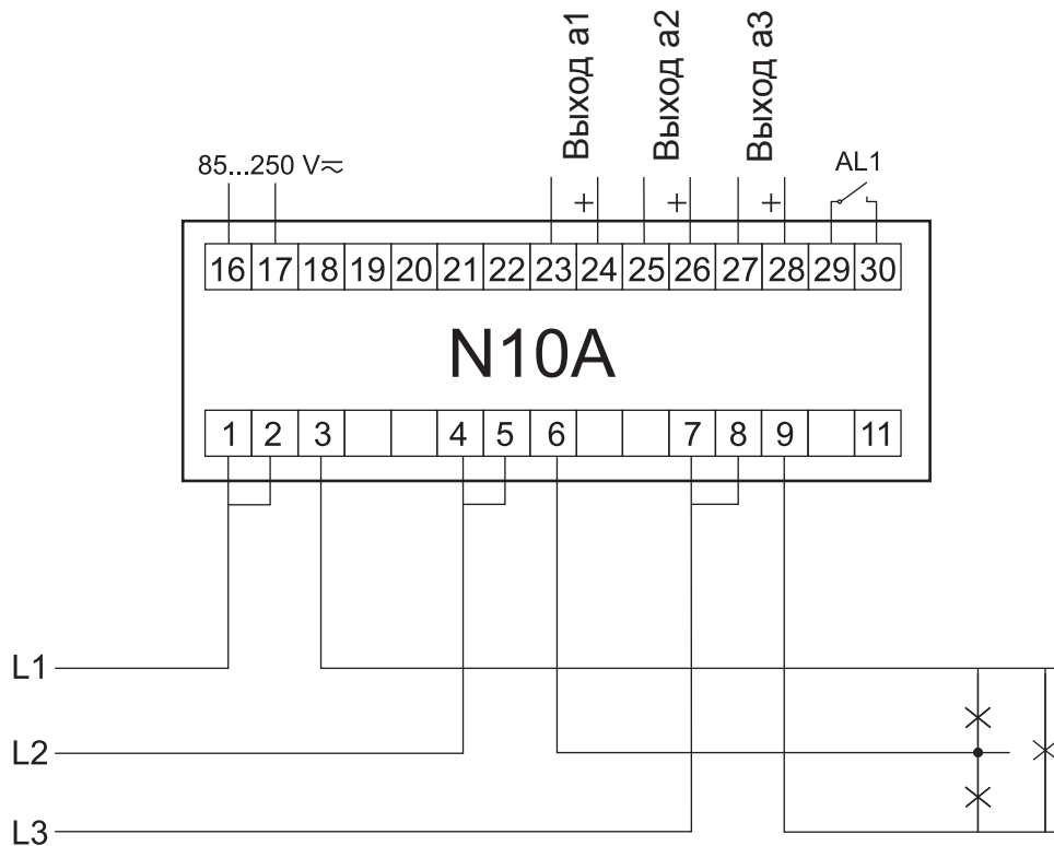
Прямое измерение в 3-проводной сети
