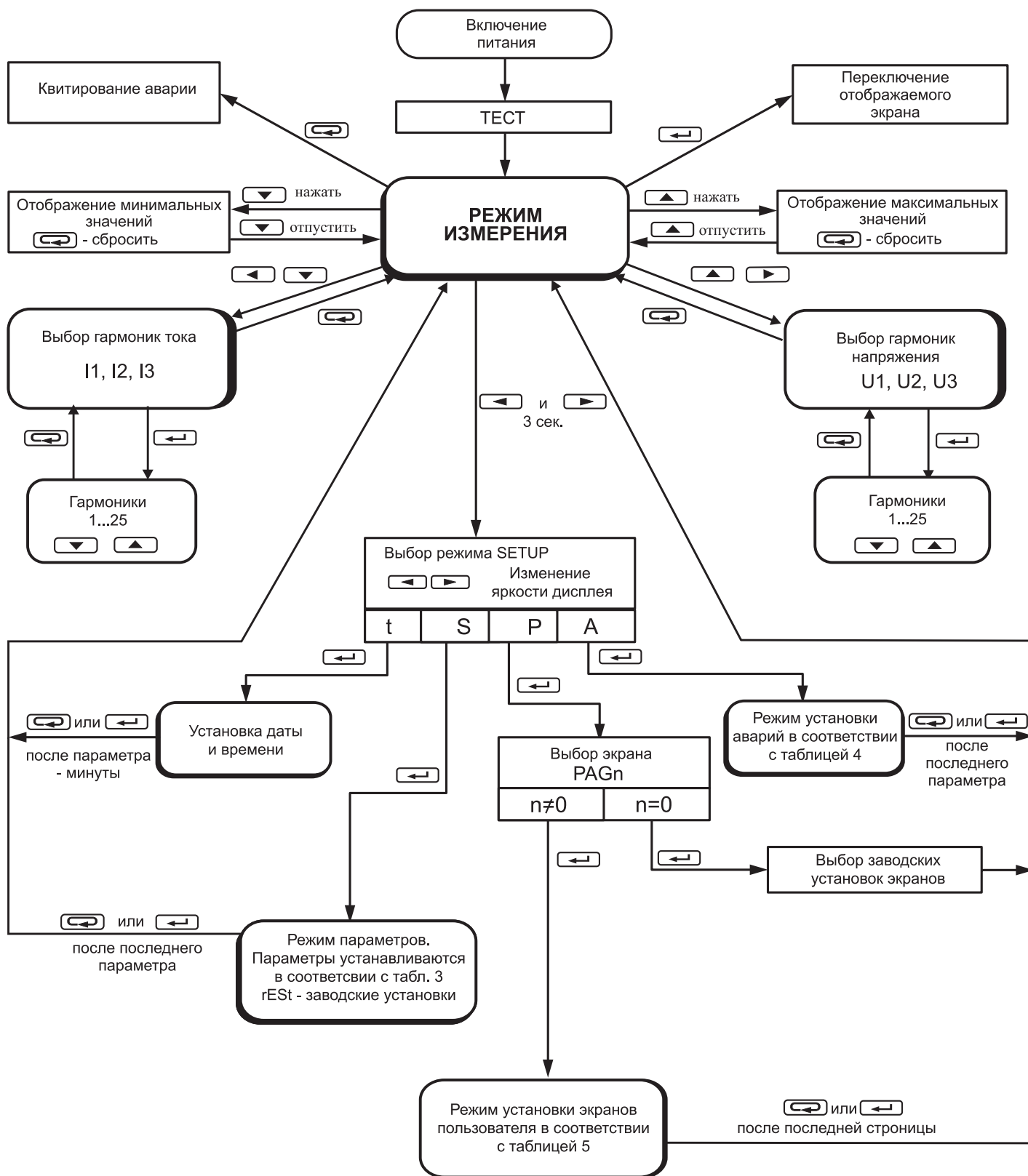
Рис.6. Режимы работы анализатора N10A.
