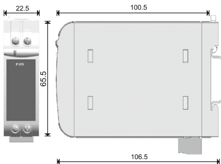
Rys. 7. Wymiary przetwornika.
