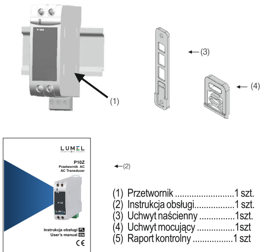
Rys. 2: Zestaw przetwornika.
