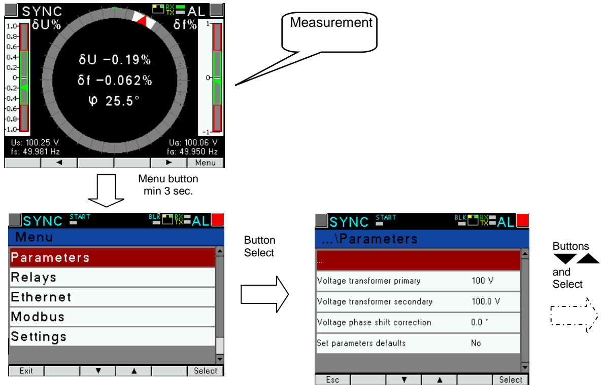
Fig.12, Screens of Parameter group
