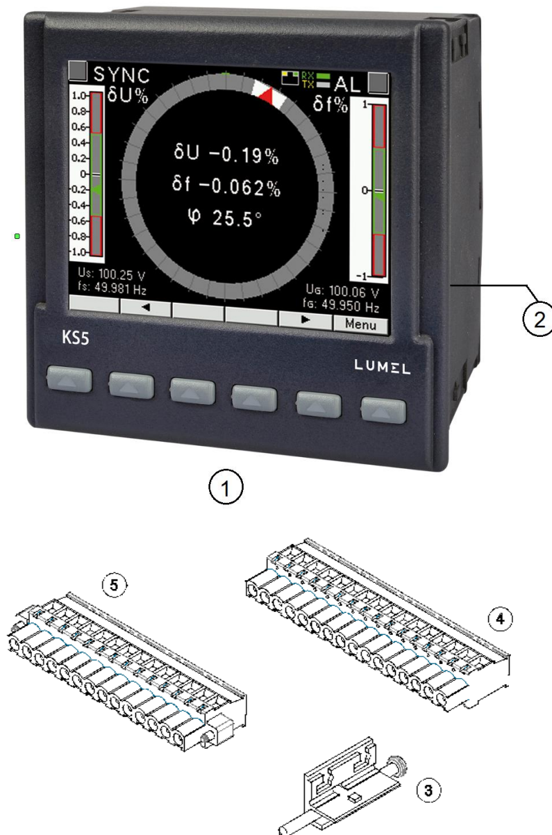
Fig.1, Meter set
