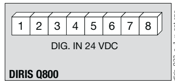
DIRIS Q800 1-2: optocoupler input 1 3-4: optocoupler input 2 5-6: optocoupler input 3 7-8: optocoupler input 4
