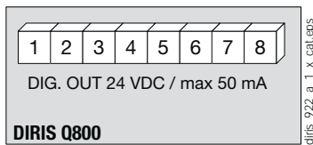
DIRIS Q800 1-2: optocoupler output 1 3-4: optocoupler output 2 5-6: optocoupler output 3 7-8: optocoupler output 4
