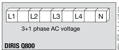
DIRIS Q800 L1, L2, L3, L4, N: voltage inputs
